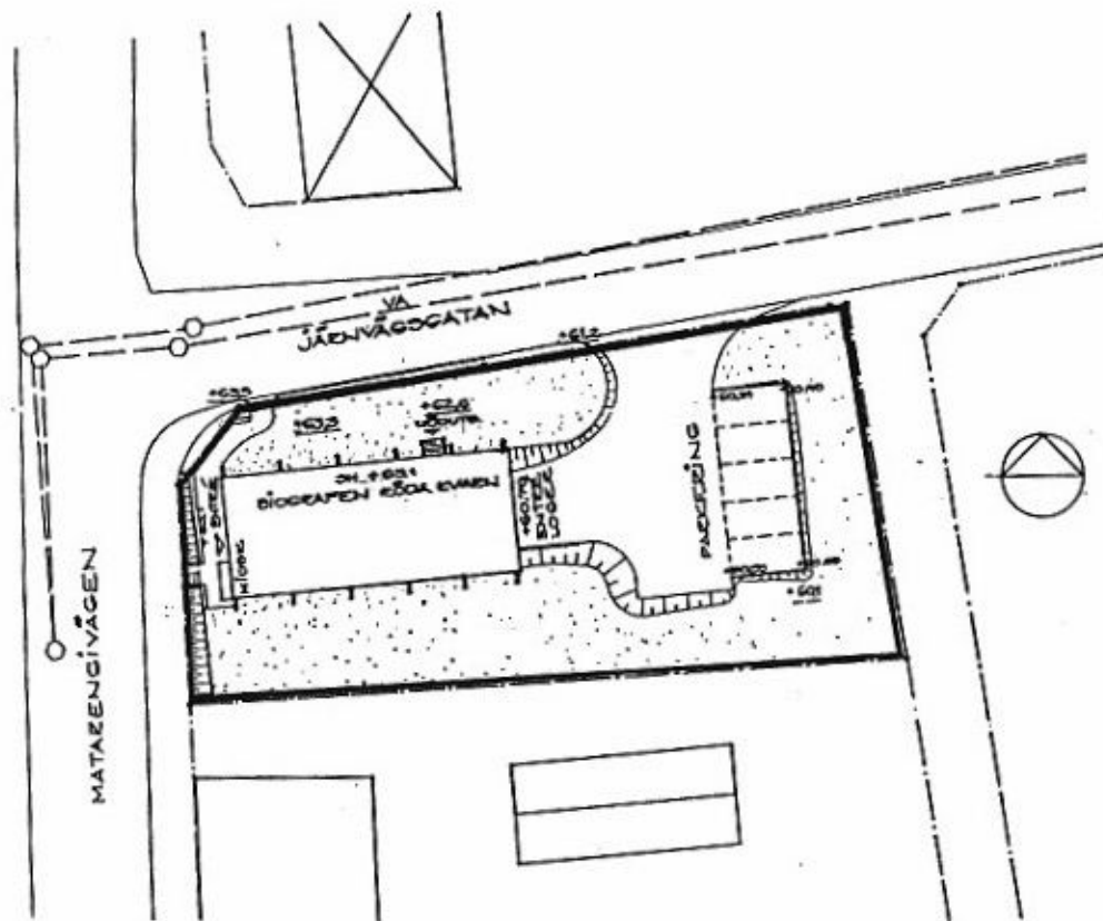
SITUATIONSPÅN 1:200 FASTIGHETEN MATARENGI 11116
