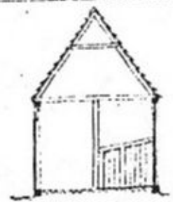
SEKT. D-D
