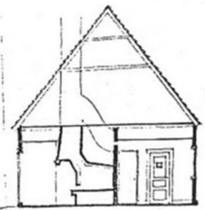
SEKT. B-B
