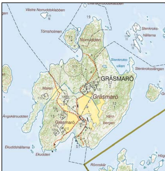
Skärgårdskarta över Gräsmarö
