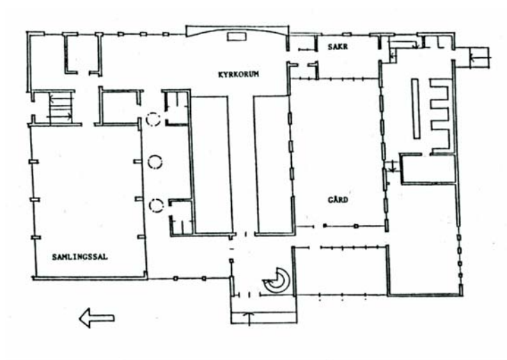
Planritning hämtad ur Nya svenska kyrkor. Kyrkorummet i mitten, flankerat av församlingshem till vänster och pastorsexpedition till höger.
