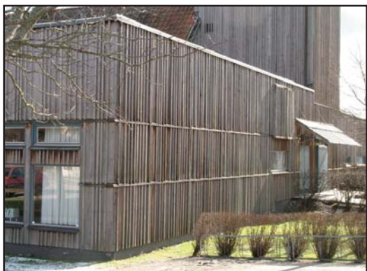
Fasadbeklädnaden av tryckimpregnerad furu består av lockbräder med olika bredd och kraftiga läkt, vilket skapar en viss rytm.
