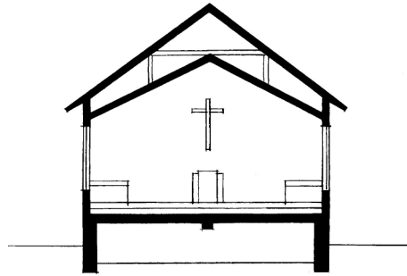
Sektion
