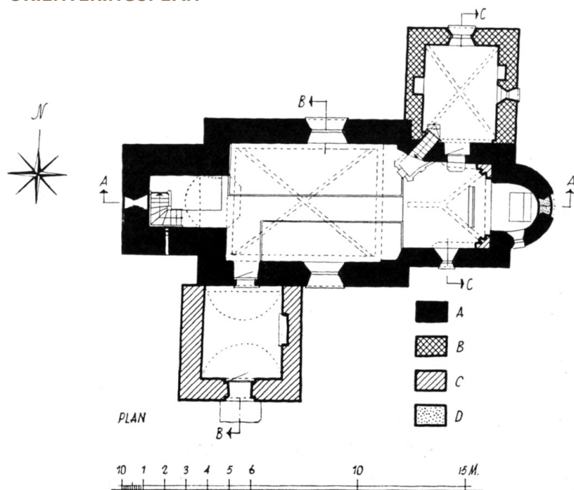
Plan av kyrkan mot norr. Uppmätt av J. Söderberg 1948. Sveriges kyrkor.
