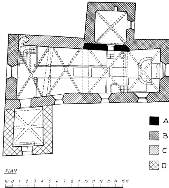
Plan av Hammarby kyrka mot norr. Uppmätning från 1921, kompletterad 1948. Ur Sveriges kyrkor.
