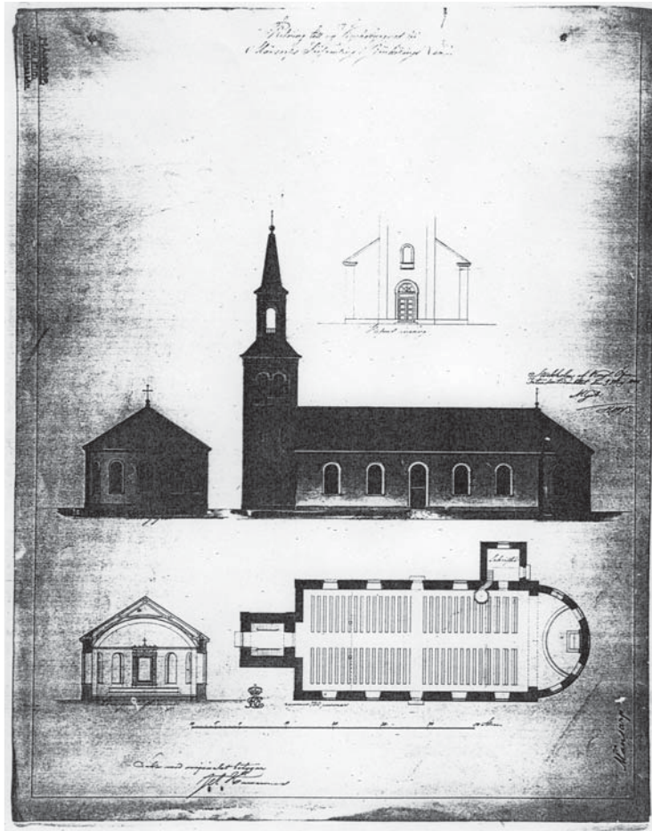
Arkitekt J A Hawermans slutliga ritning till kyrka för Månsarp. ATA.
