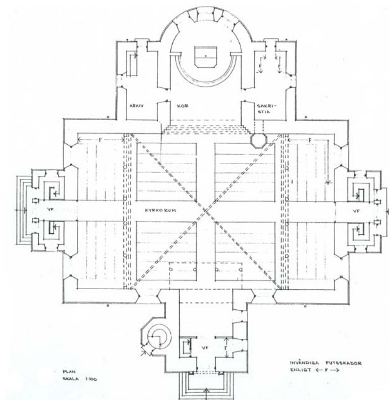
Uppmätning utförd av arkitekt Johannes Dahl 1969.
