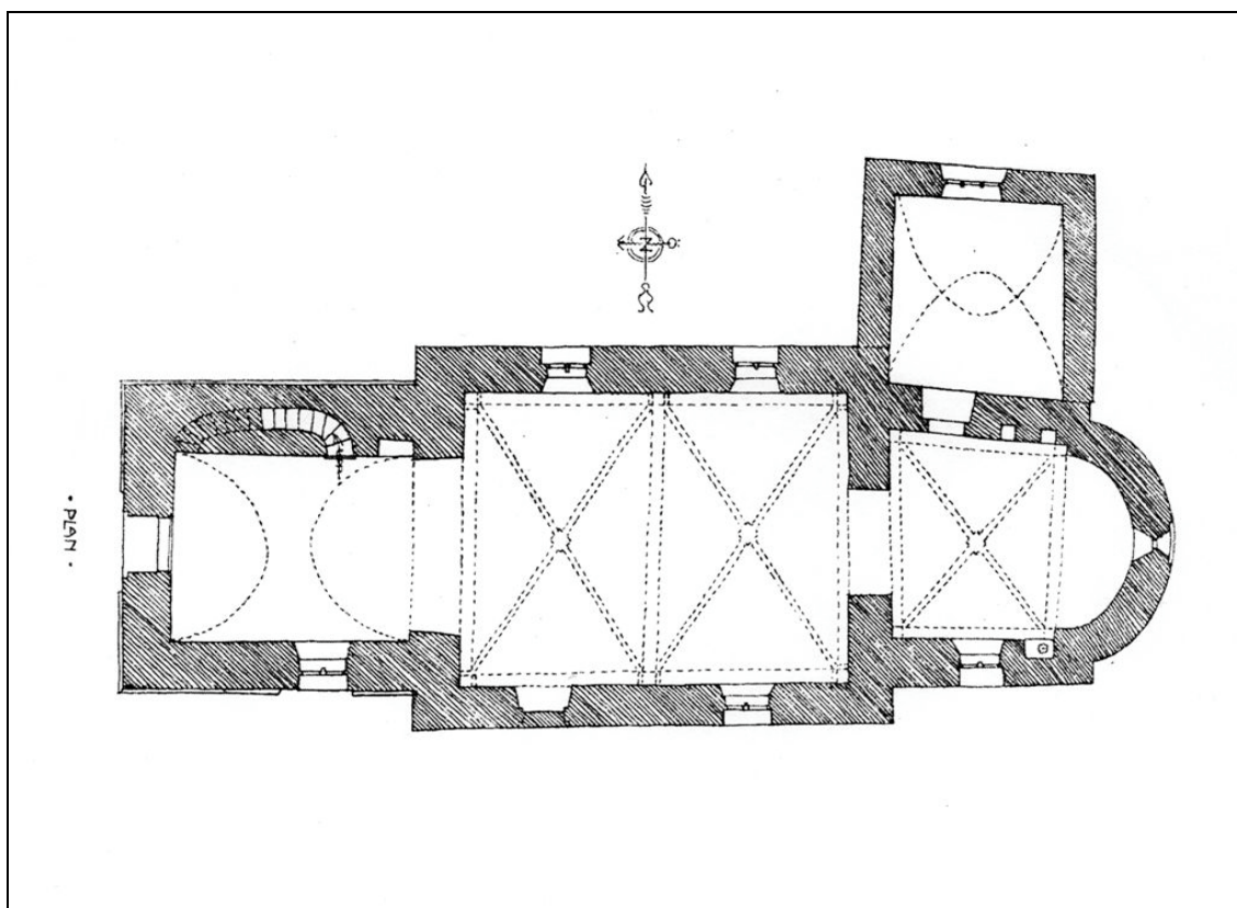
Plan över Kumlaby kyrka upprättad av Anders Roland 1908.
