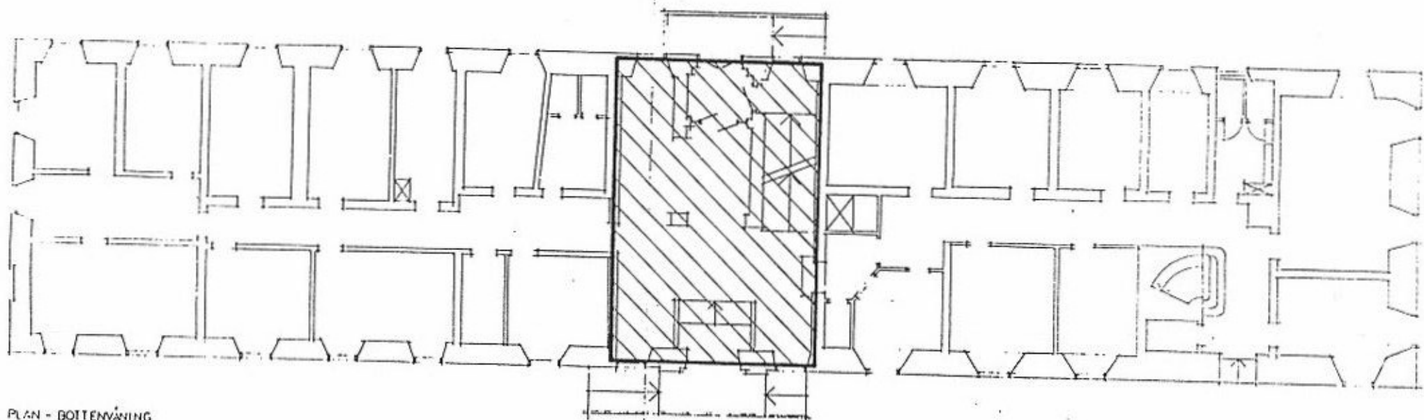
PLAN - BOTTENVÅNING
