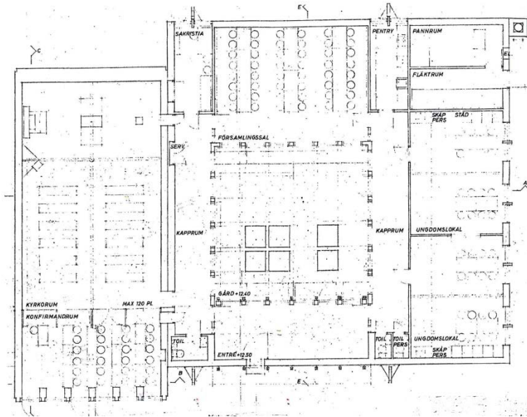
Plan över Hyllinge småkyrka. Öster är uppåt på ritningen.
