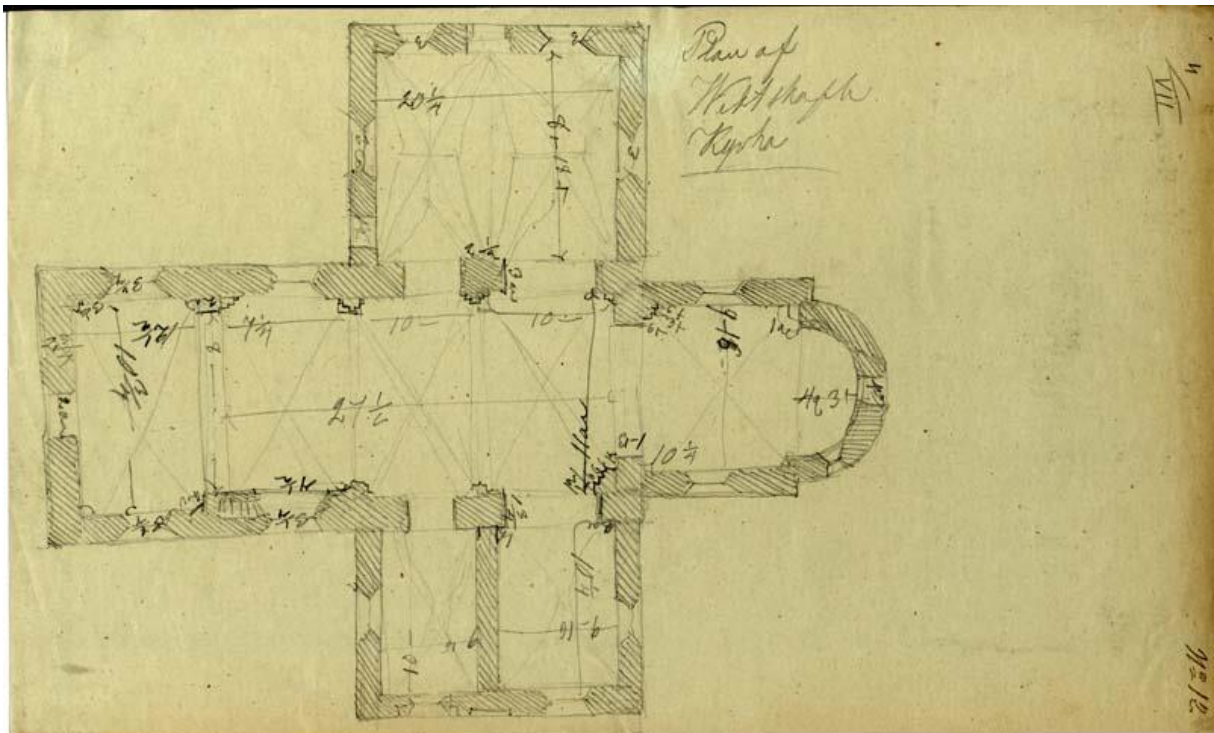
Planskiss av kyrkan utförd av Nils Månsson Mandelgren, 1865. Observera den äldre torntrappan i söder. Bilden är hämtad från Mandelgrenska samlingen, Lunds universitet.
