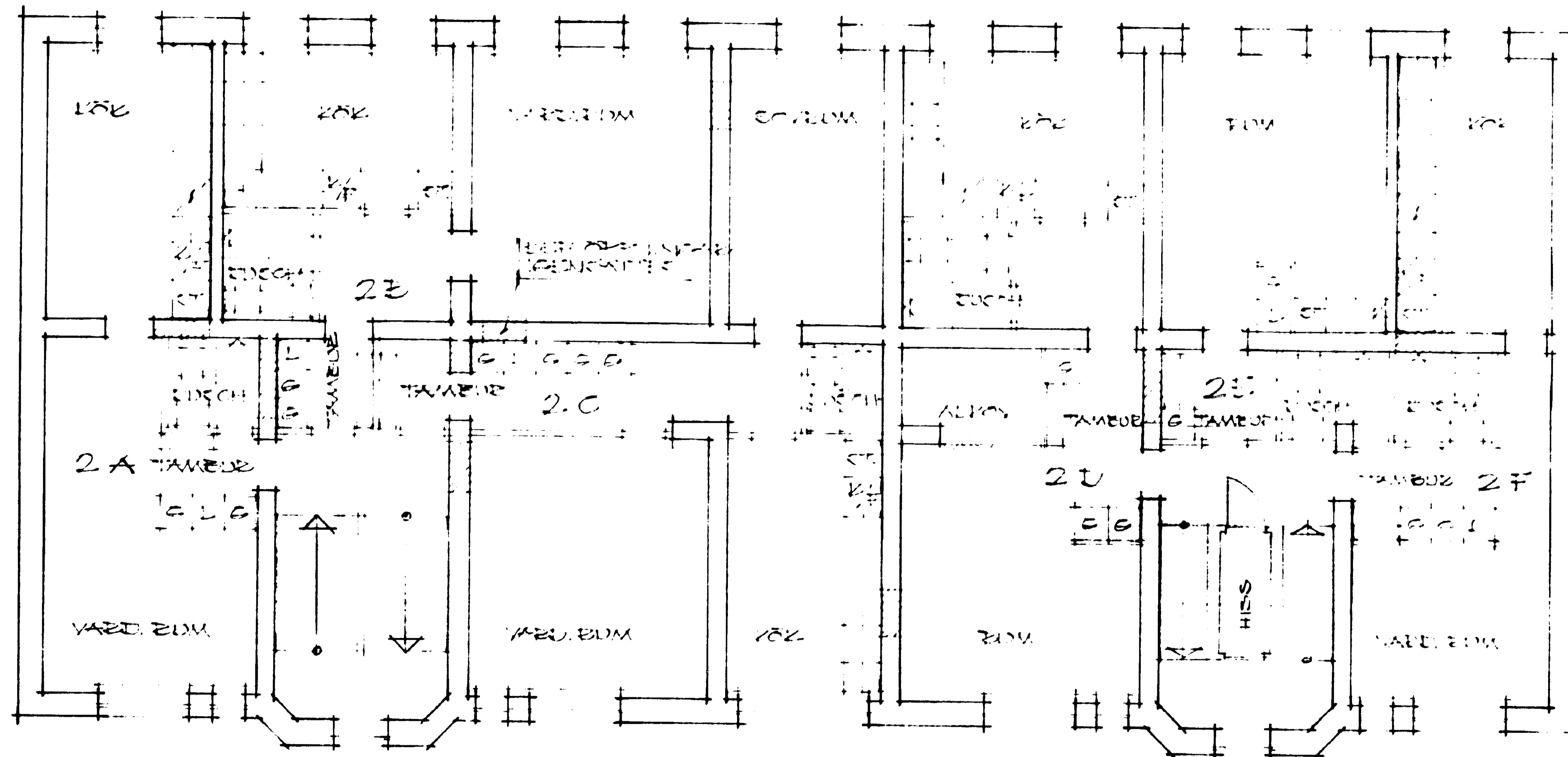
VÄN. 2 TRAFFOR 1:100
