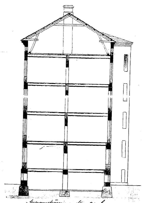
Sannskärning för a-b
