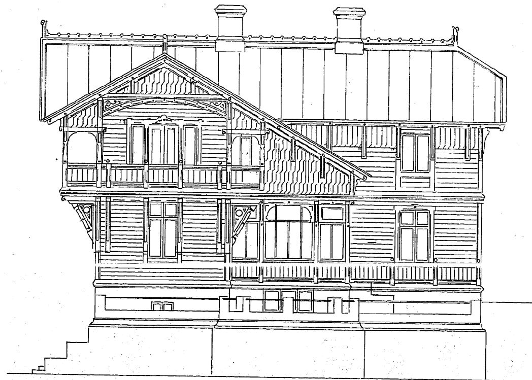
FAÇADE MOT VESTER
