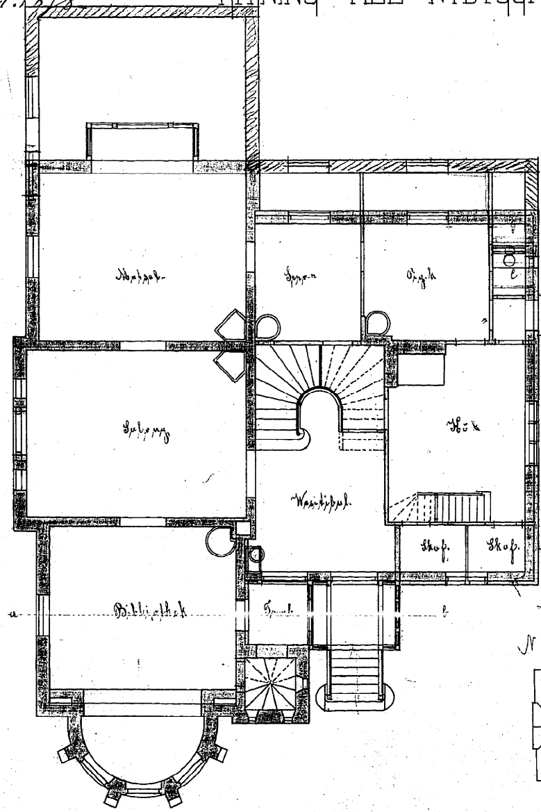
PLAN AF 1 ste VÅNINGEN
