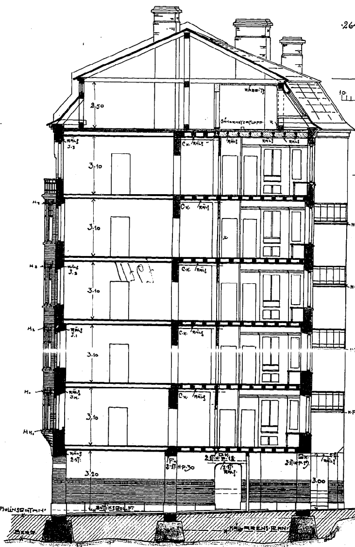
SEKTION A.B.
