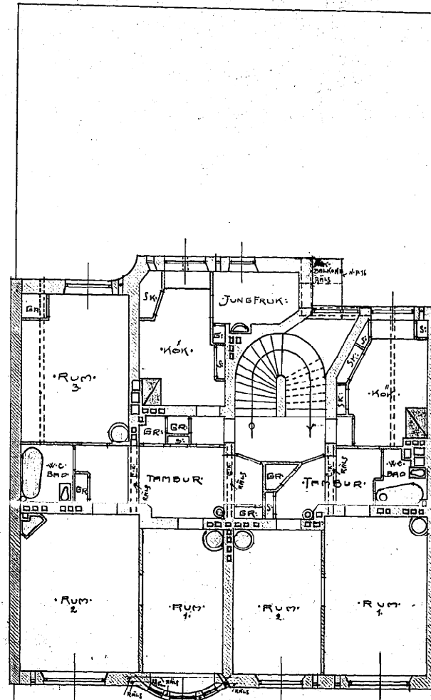
4 DE VÅNINGENS PLAN
