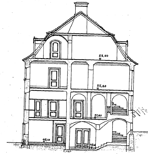
Tvärsektion.
