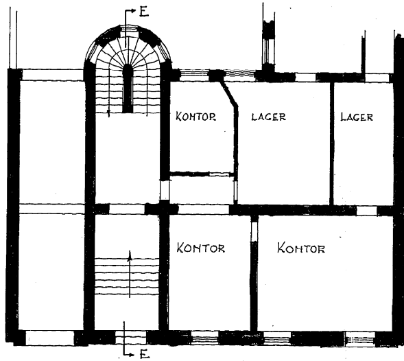
FÖRSTA VÅNINGEN.
