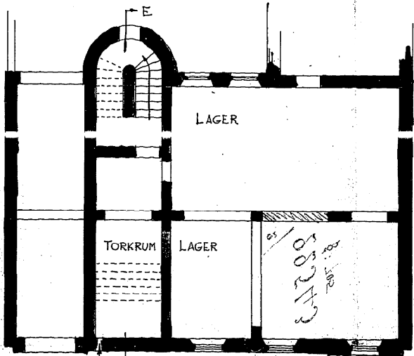
KÄLLAREN.
