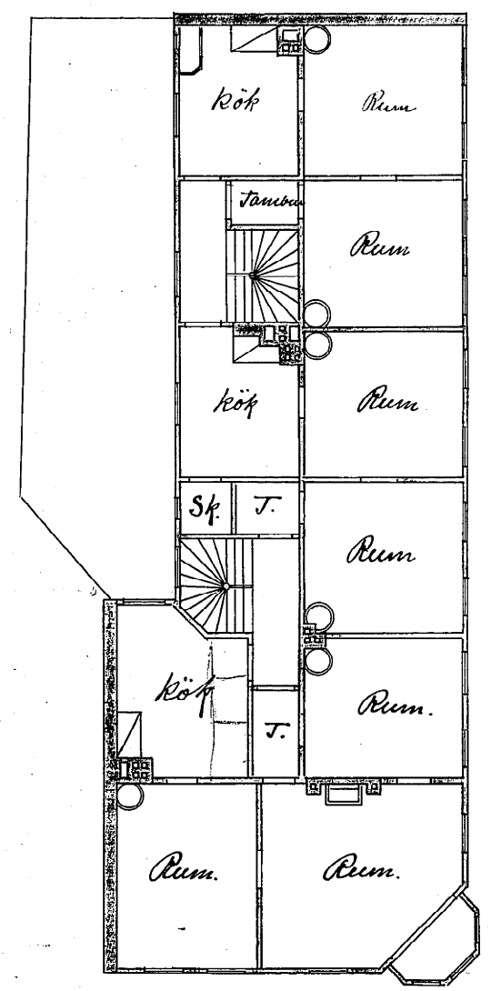
2:a Våningen
