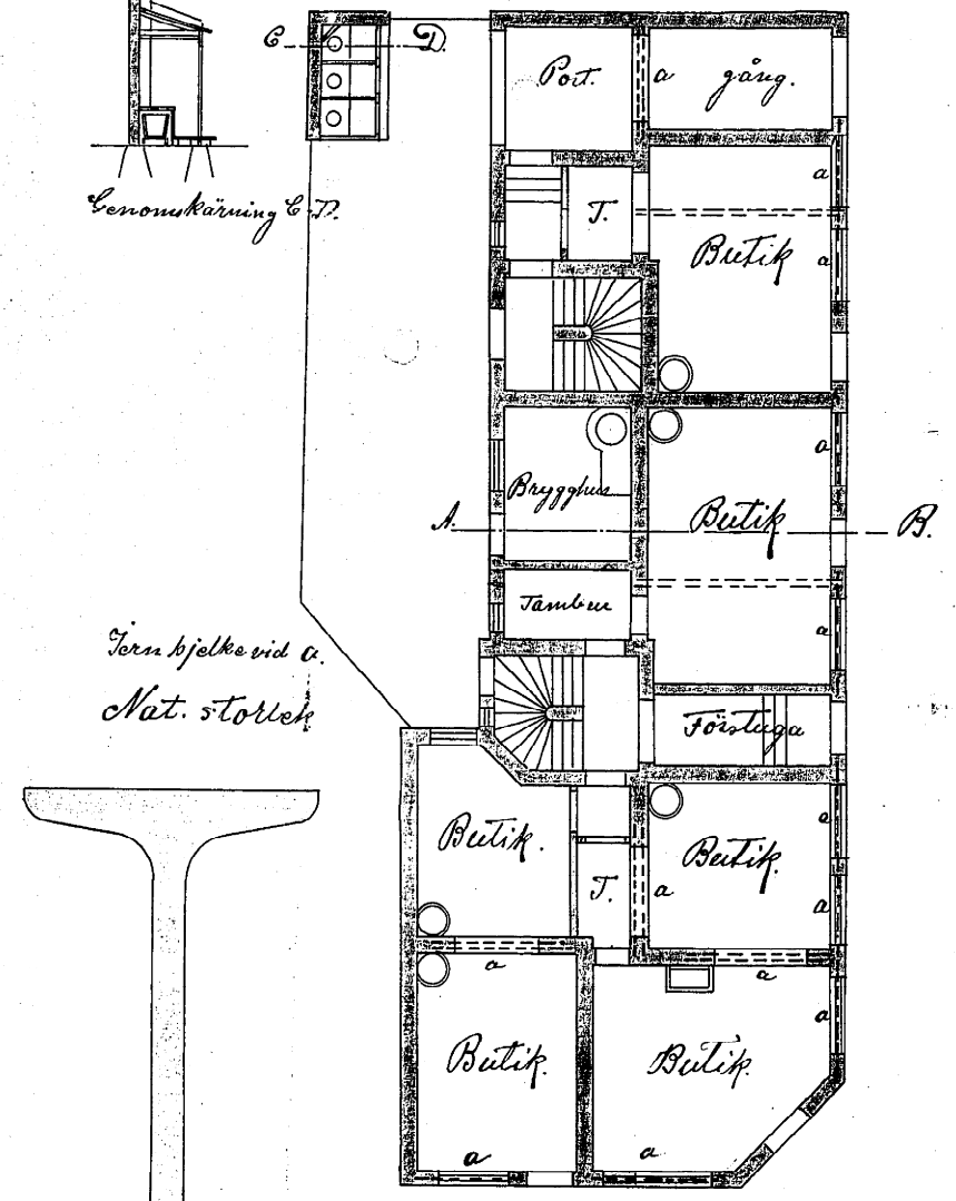
Källaren
