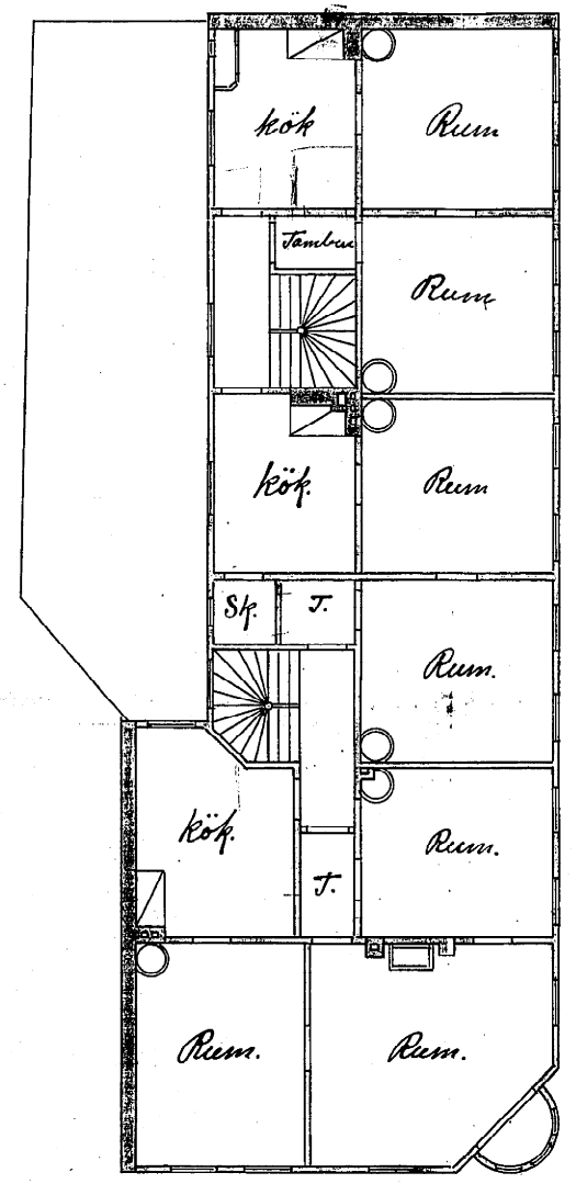
1:a Våningen
