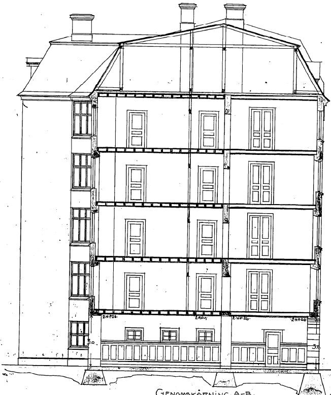
GENOMSKÄRNING A-B
