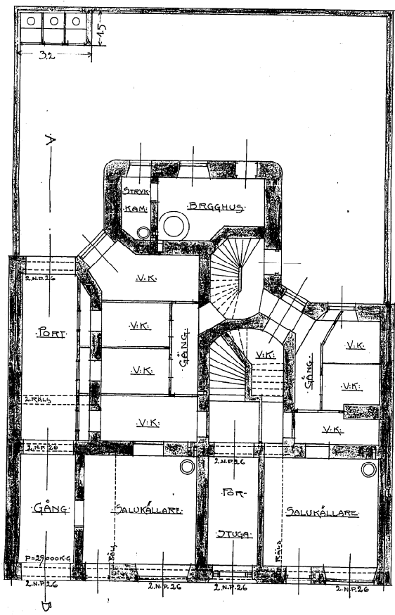
PLAN AF KÄLLAREN.
