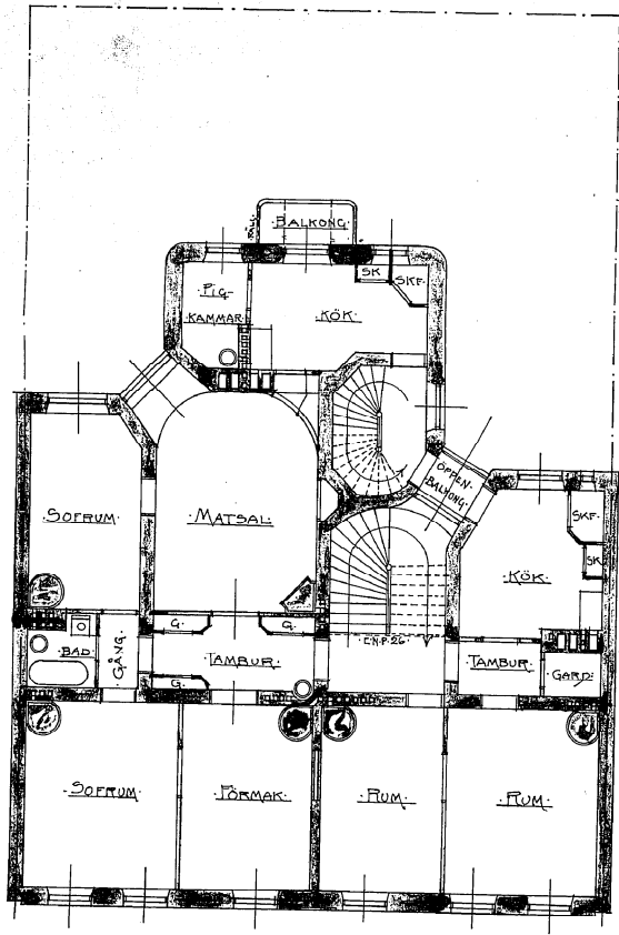
PLAN AF 3 DE VÅNINGEN.
