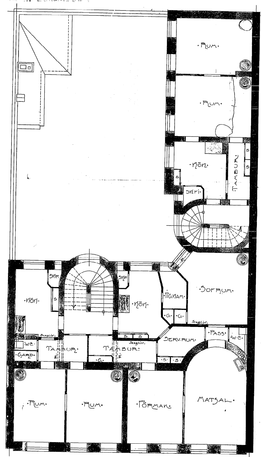
•FÖRSTA VÅNINGEN.
