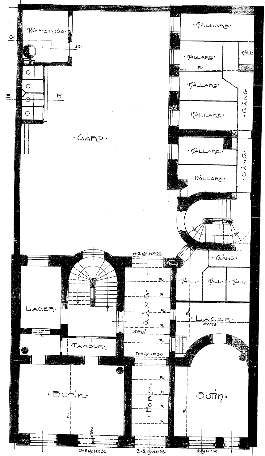
•KÄLLAREN.
