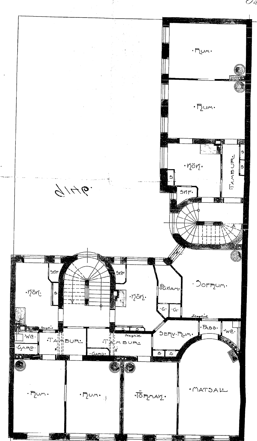
•ANDRA VÅNINGEN.
