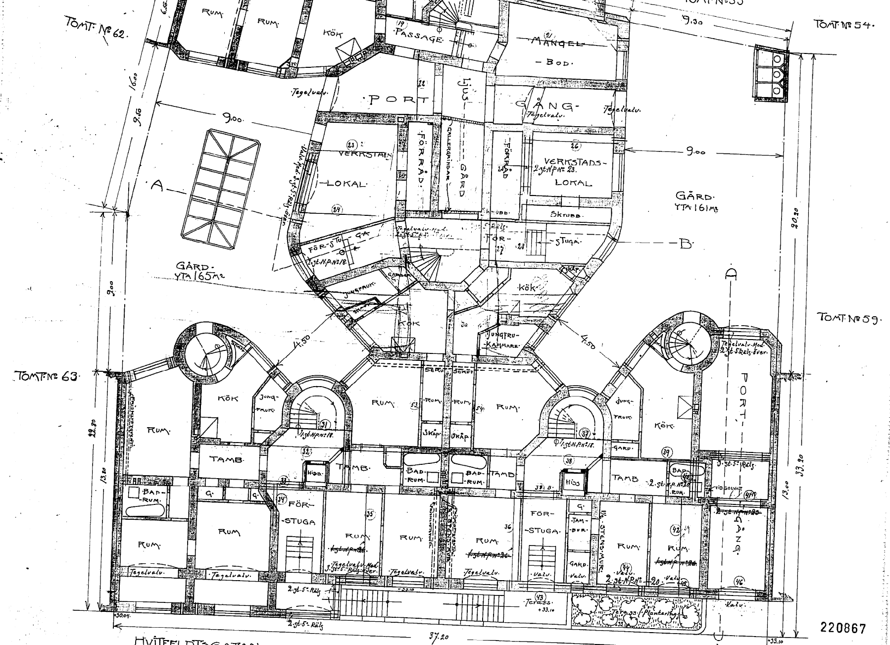
HVITFELDTGATAN. 1 ST VÅNINGEN OCH SITUATIONSPLAN.
