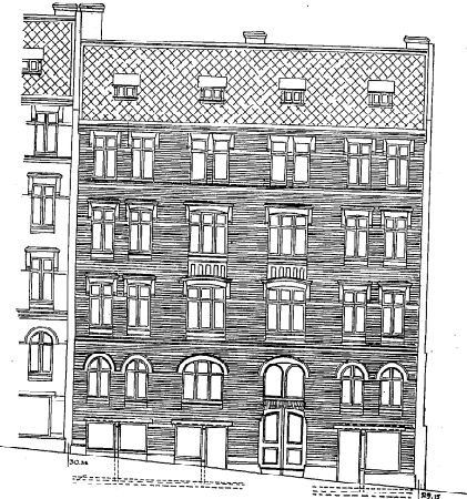
Fasad mot Kungshöjdgatan
