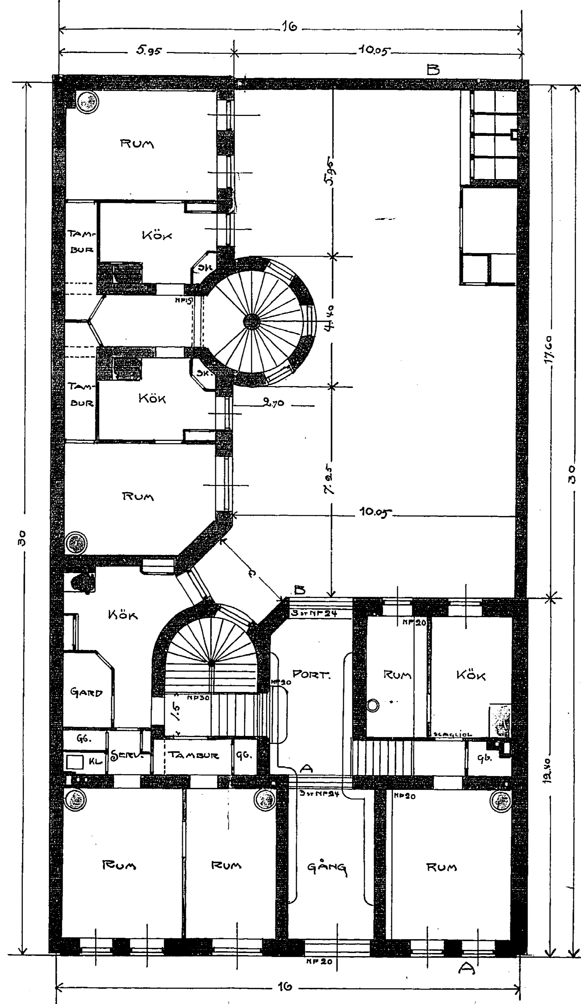
PLAN AF 1 sta VÅNINGEN
