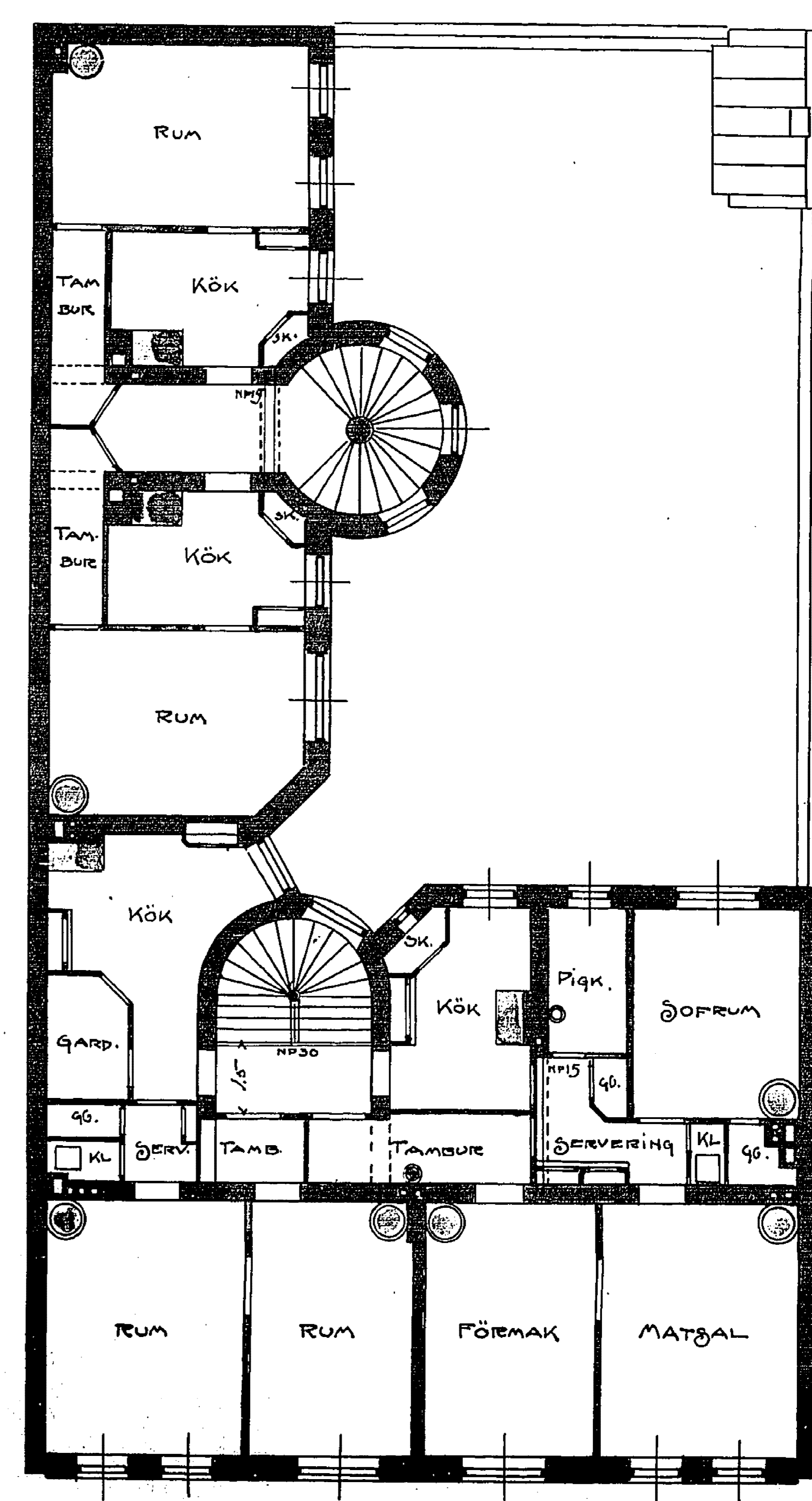
PLAN AF 2 dra VÅNINGEN
