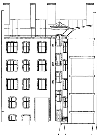
FASAD MOT VÄST
