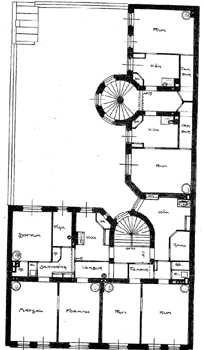
PLAN AF 2 STE VÅNINGEN
