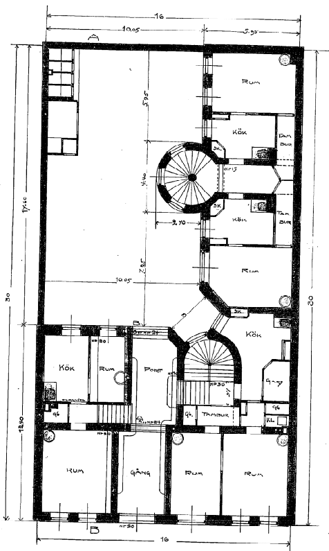
PLAN AF 1 STE VÅNINGEN
