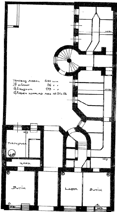
PLAN AF KÄLLAREN
