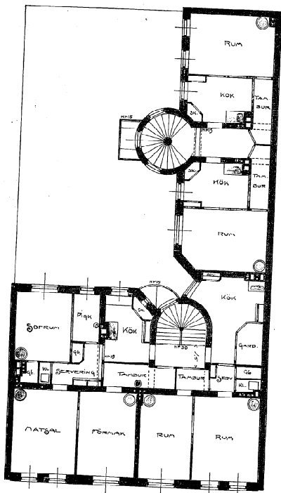
PLAN AF 3 DE VÅNINGEN
