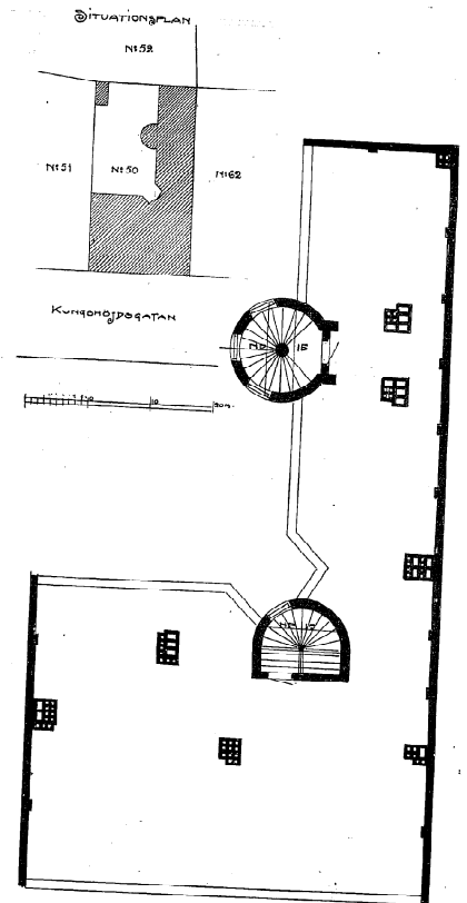
PLAN AF VINDEN
