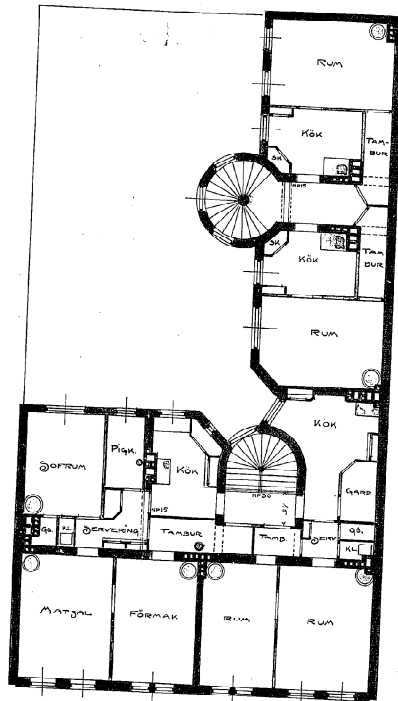
PLAN AF 4 DE VÅNINGEN
