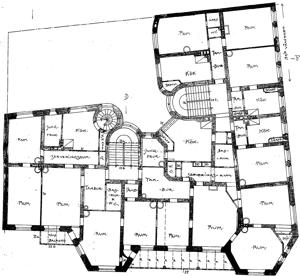
2DRA VÅNINGEN
