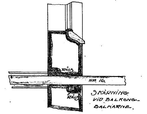
SKÄRNING GENOM AFTRÅDET
