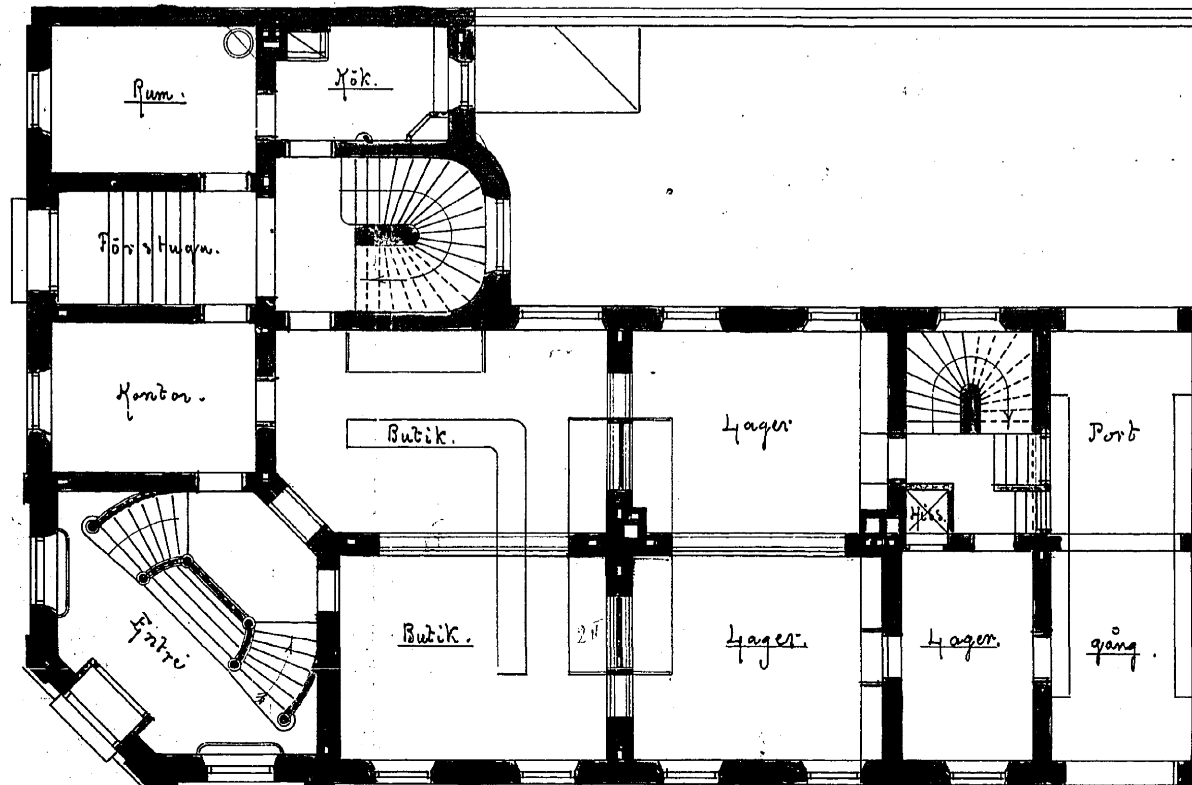
Plan af Bottenwåningen.
