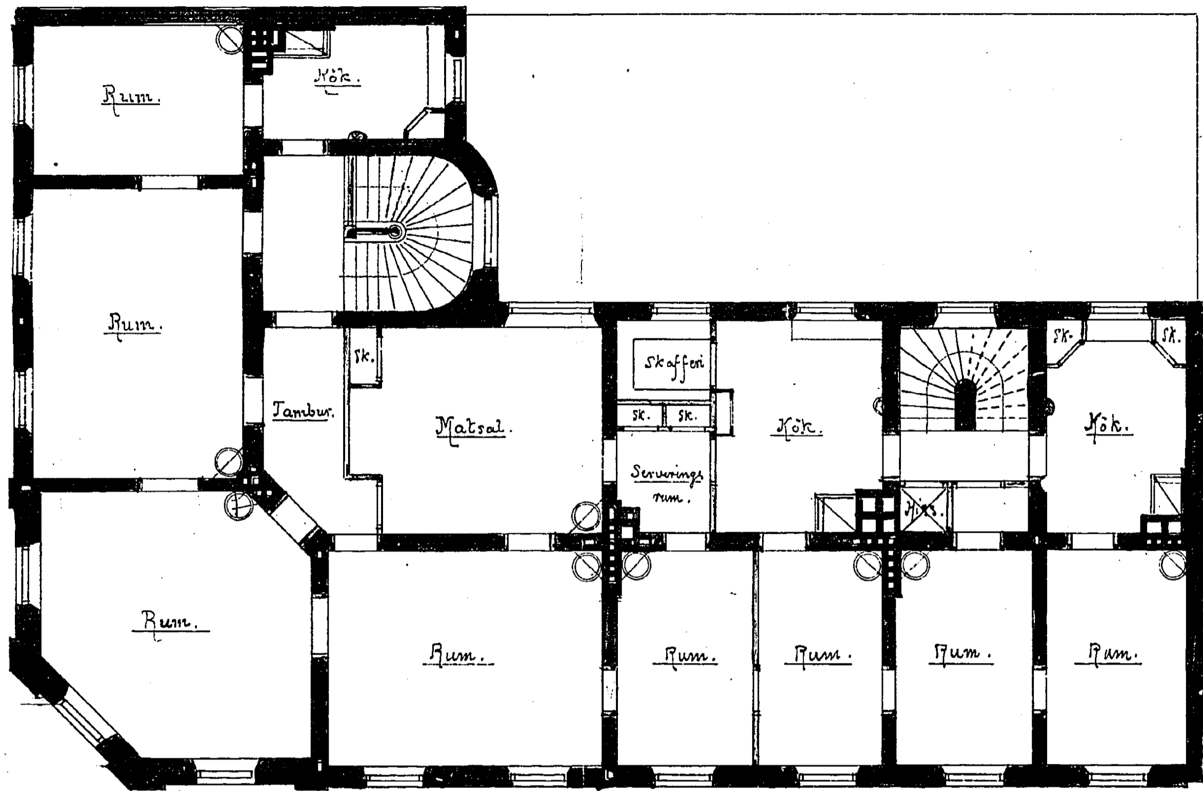
Plan af 3 de Wåningen.
