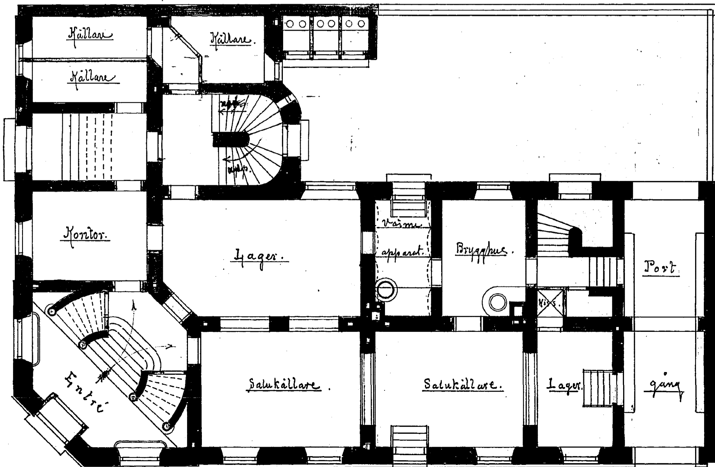
Plan af Källaren
