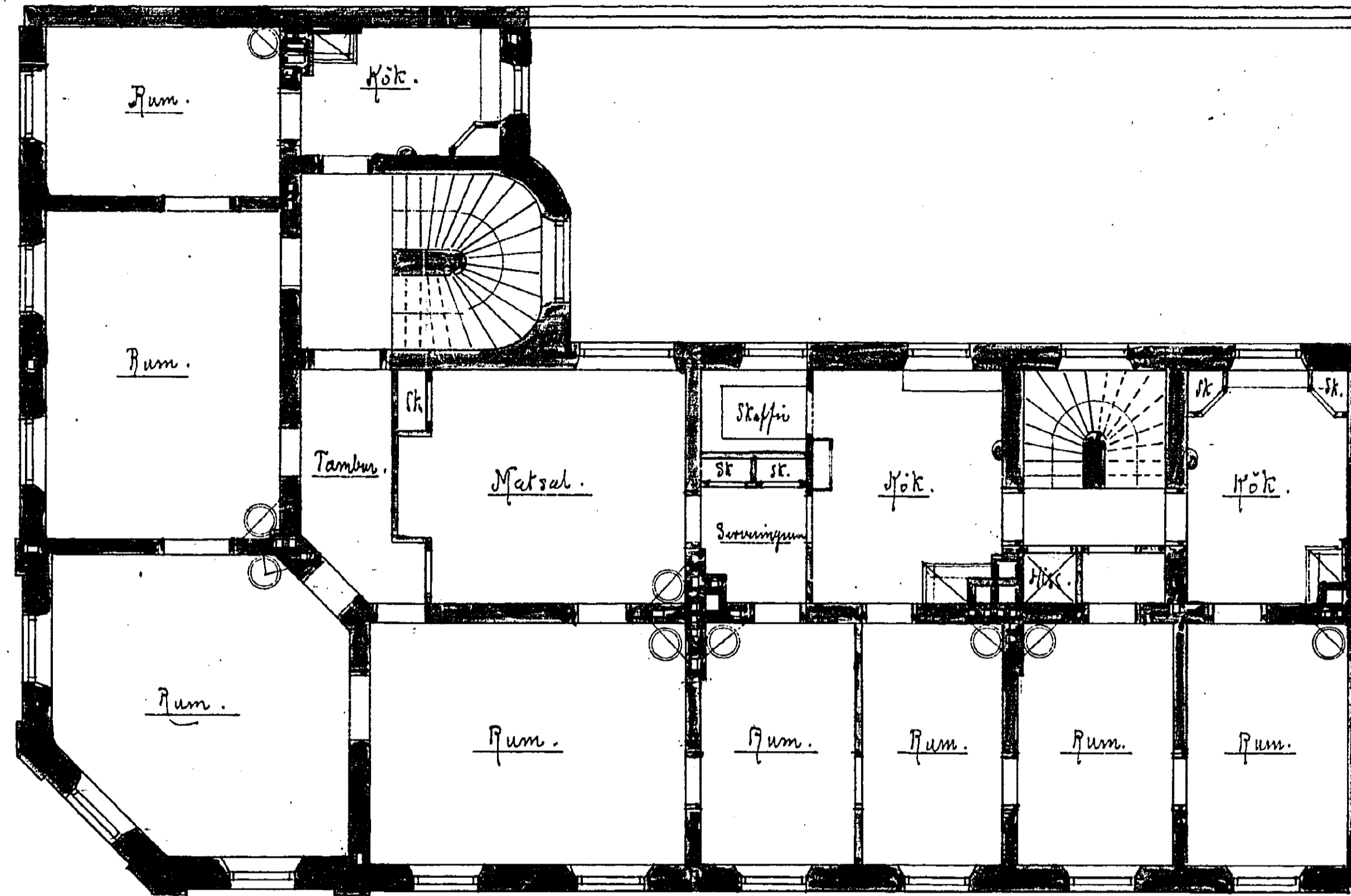
Plan af 2 de Wåningen.
