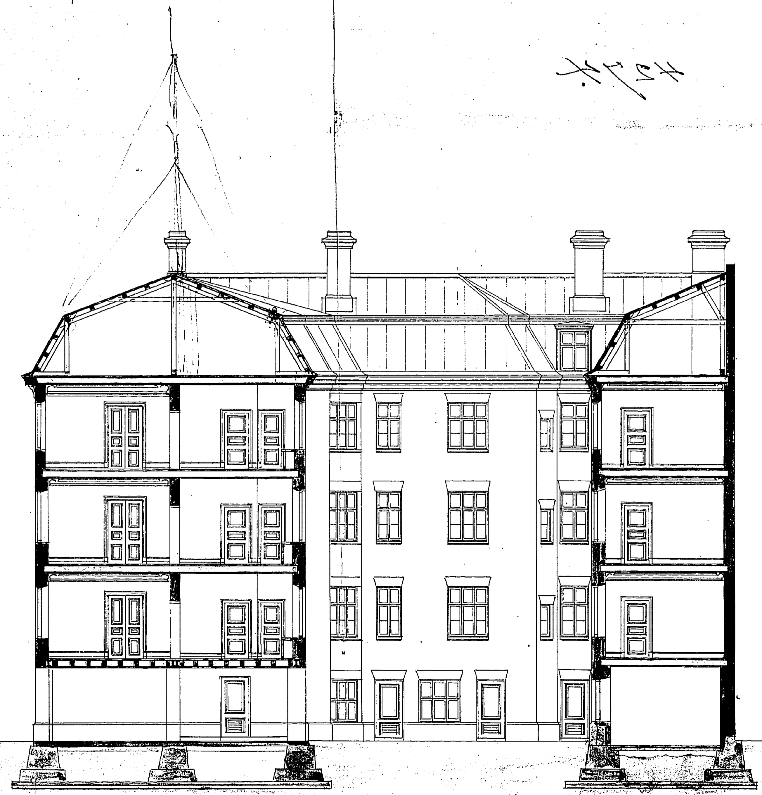
Genomskärning i A-B.
