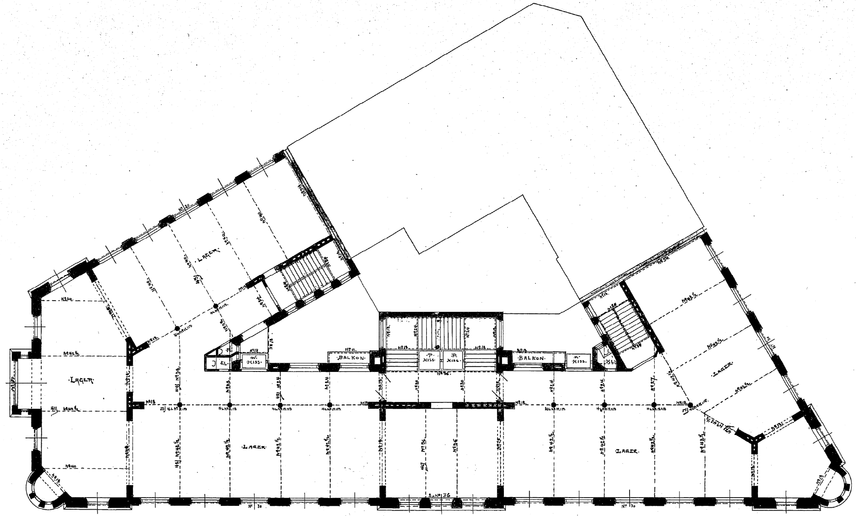
PLAN AF 3 DE VÅN.
