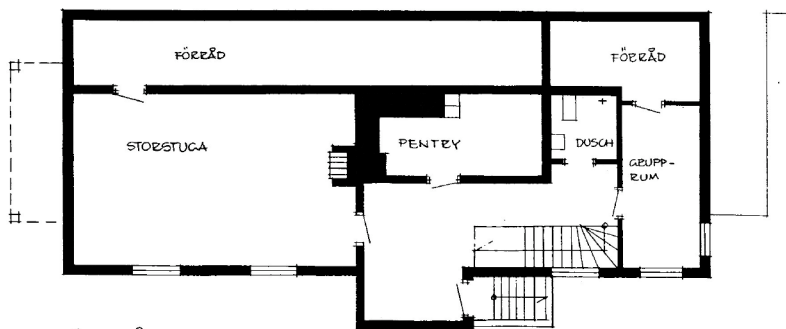
KÄLLARVÅNING
